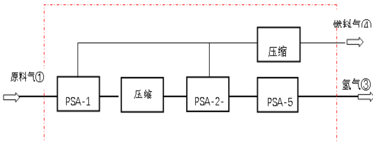
图 4.2-1 项目工艺流程图
